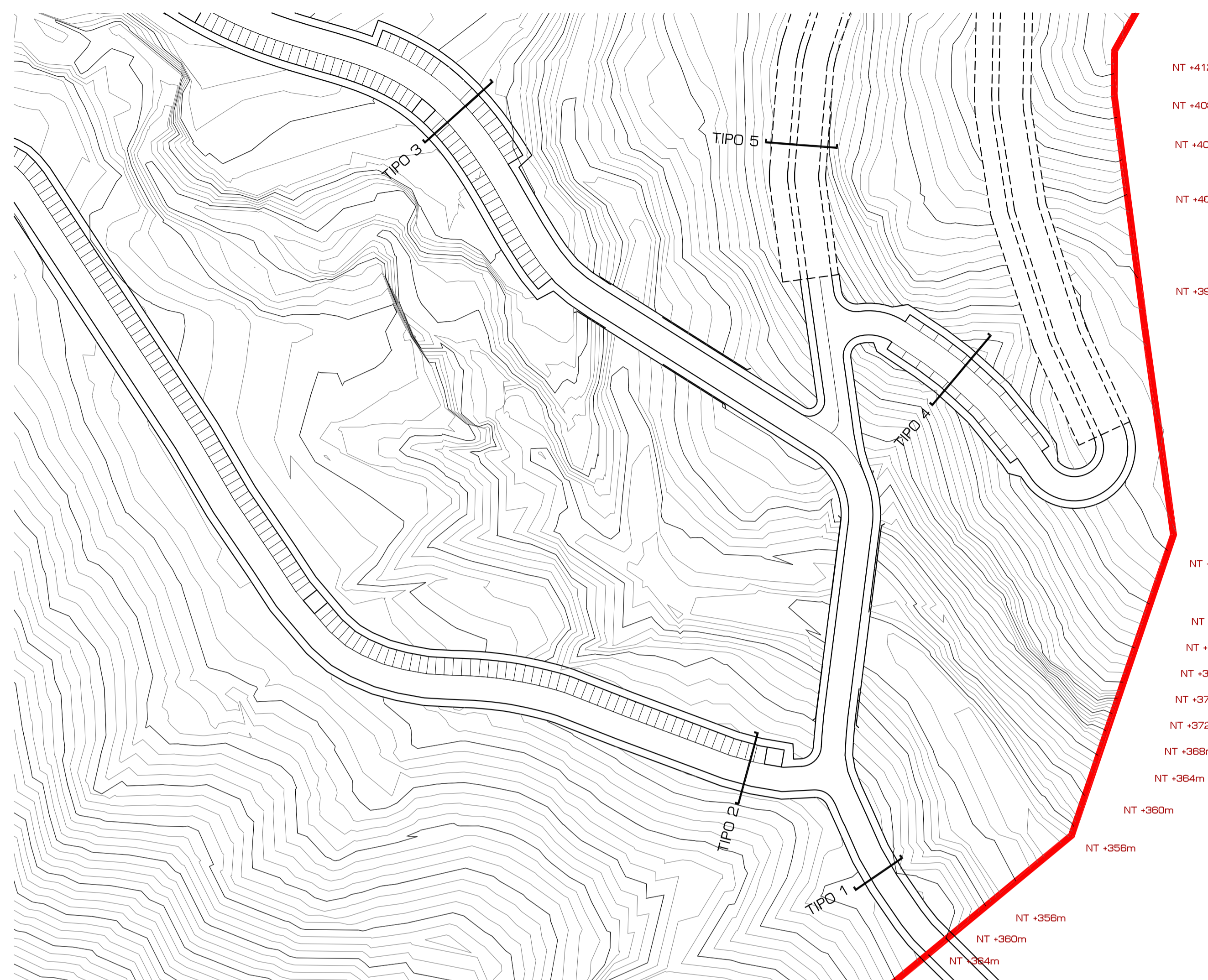
Plano llave - Secciones de viario e 1-1000
