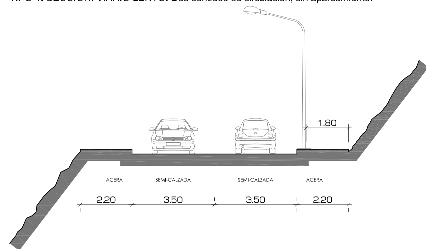
TIPO 1. SECCIÓN. VIARIO LENTO. Dos sentidos de circulación, sin aparcamiento.
