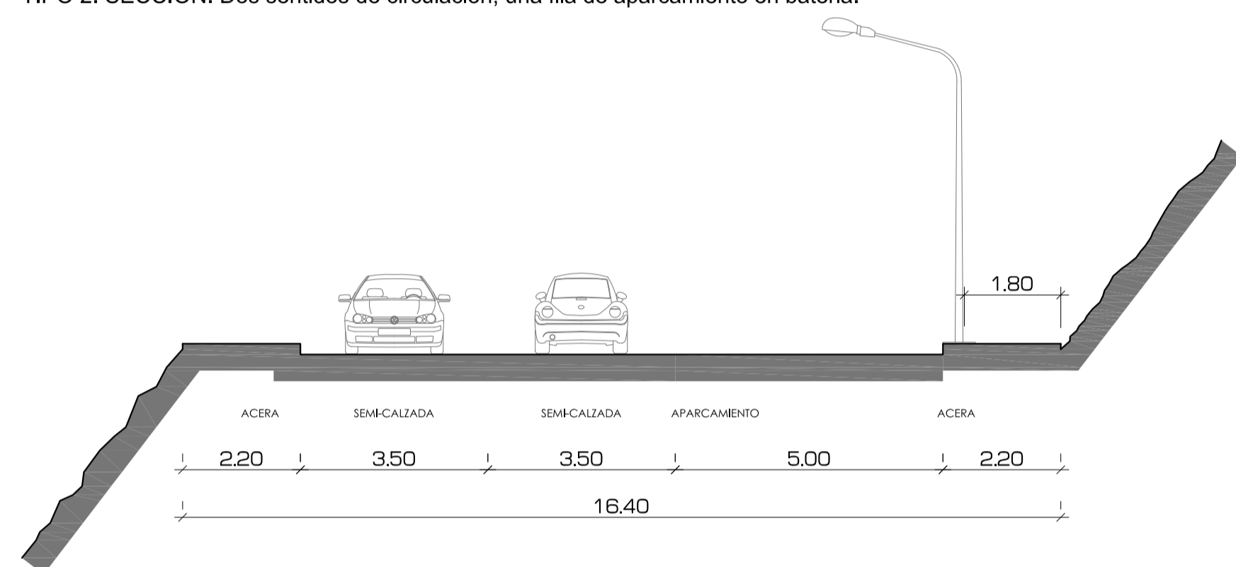
TIPO 2. SECCIÓN. Dos sentidos de circulación, una fila de aparcamiento en batería.
