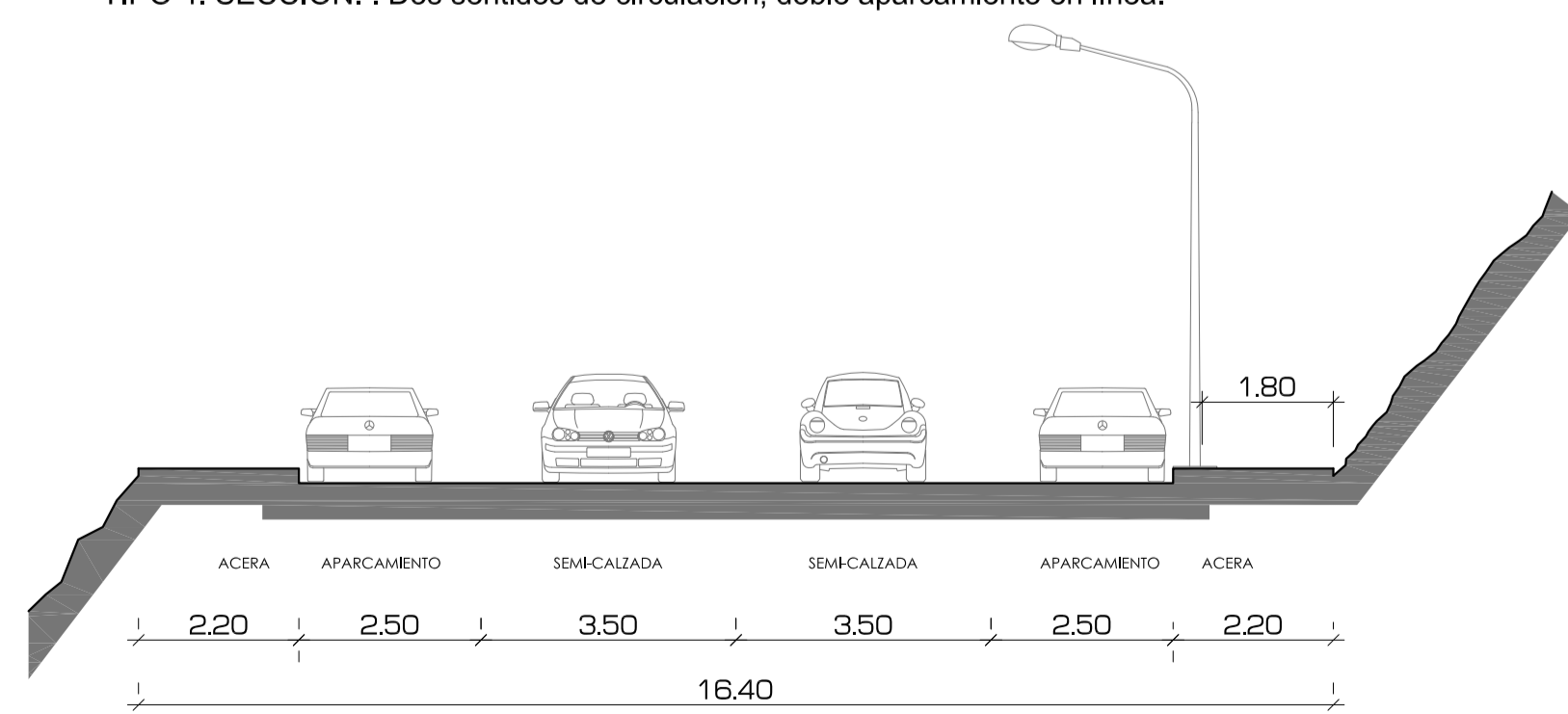
TIPO 4. SECCIÓN. . Dos sentidos de circulación, doble aparcamiento en línea.
