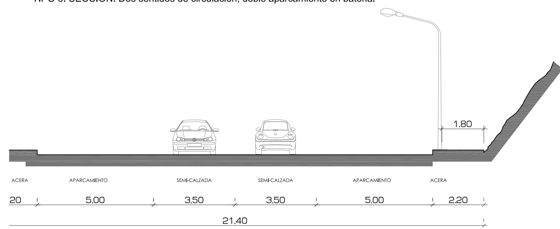
TIPO 3. SECCIÓN. Dos sentidos de circulación, doble aparcamiento en batería.
