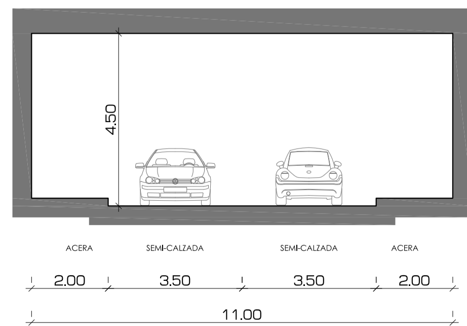
TIPO 5. SECCIÓN. VIAL SUBTERRÁNEO. Dos sentidos de circulación, sin aparcamiento.
